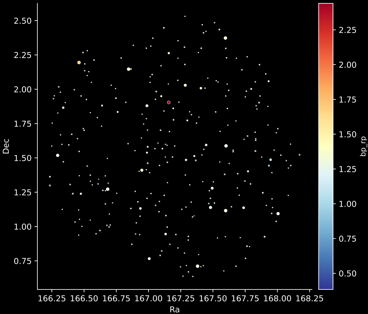
GALAH DR4 Field: [945] Stars: 284
