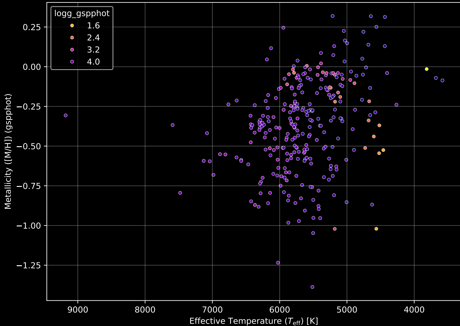
GALAH DR4 Field: [945] Stellar Population Parameters (n= 284)
